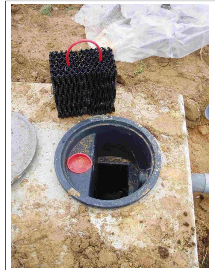
Préfiltre en plastique alvéolaire (structure de nid d'abeilles)
